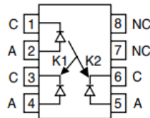
IL300
