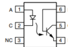
CNY17
