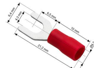
Konektor widełkowy M4 x 6,4mm izolowany Insulated crimp fork terminal M4 x 6,4mm
