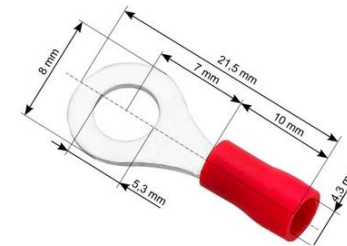
Konektor oczkowy M4 izolowany Insulated crimp ring terminal M4
